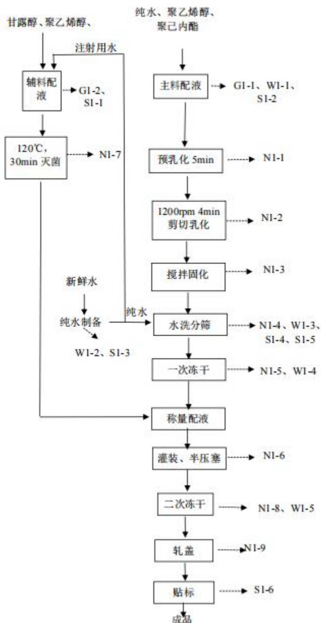
图2-2聚己内酯微球植入剂生产工艺流程图
