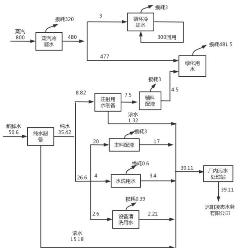
图 2-1 项目水平衡图 (t/a)
